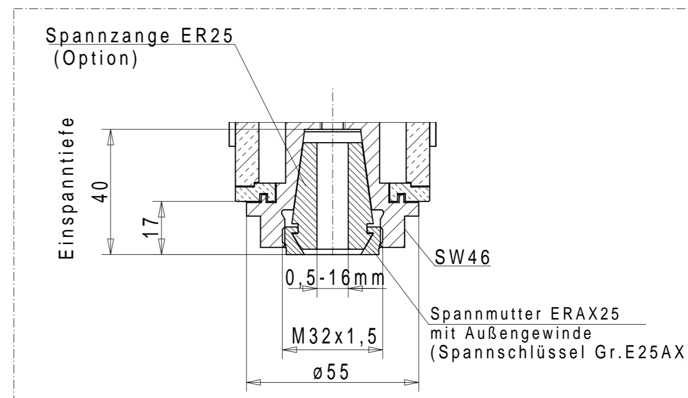
Spannzangenaufnahme HI-Q/ERAX25 mit Innengewinde
