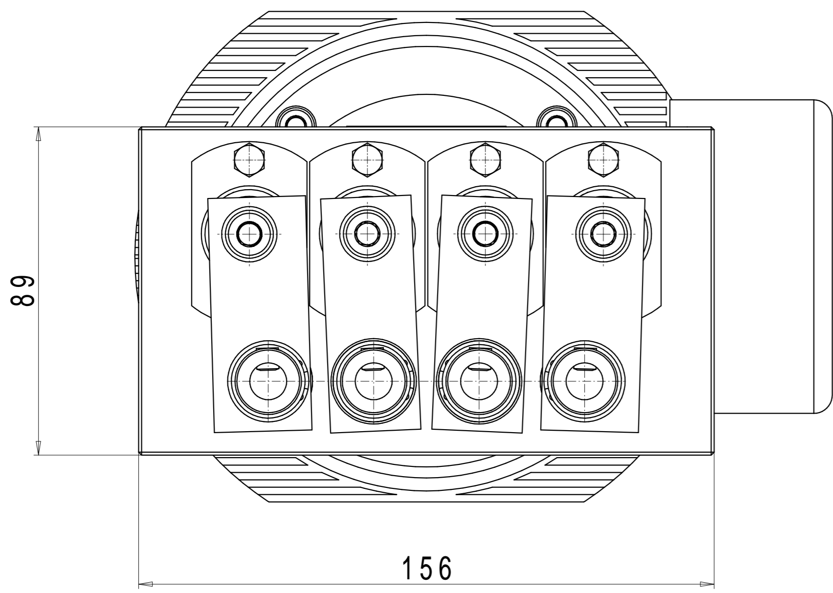
Schaftaufnahme M10 pl. RE
