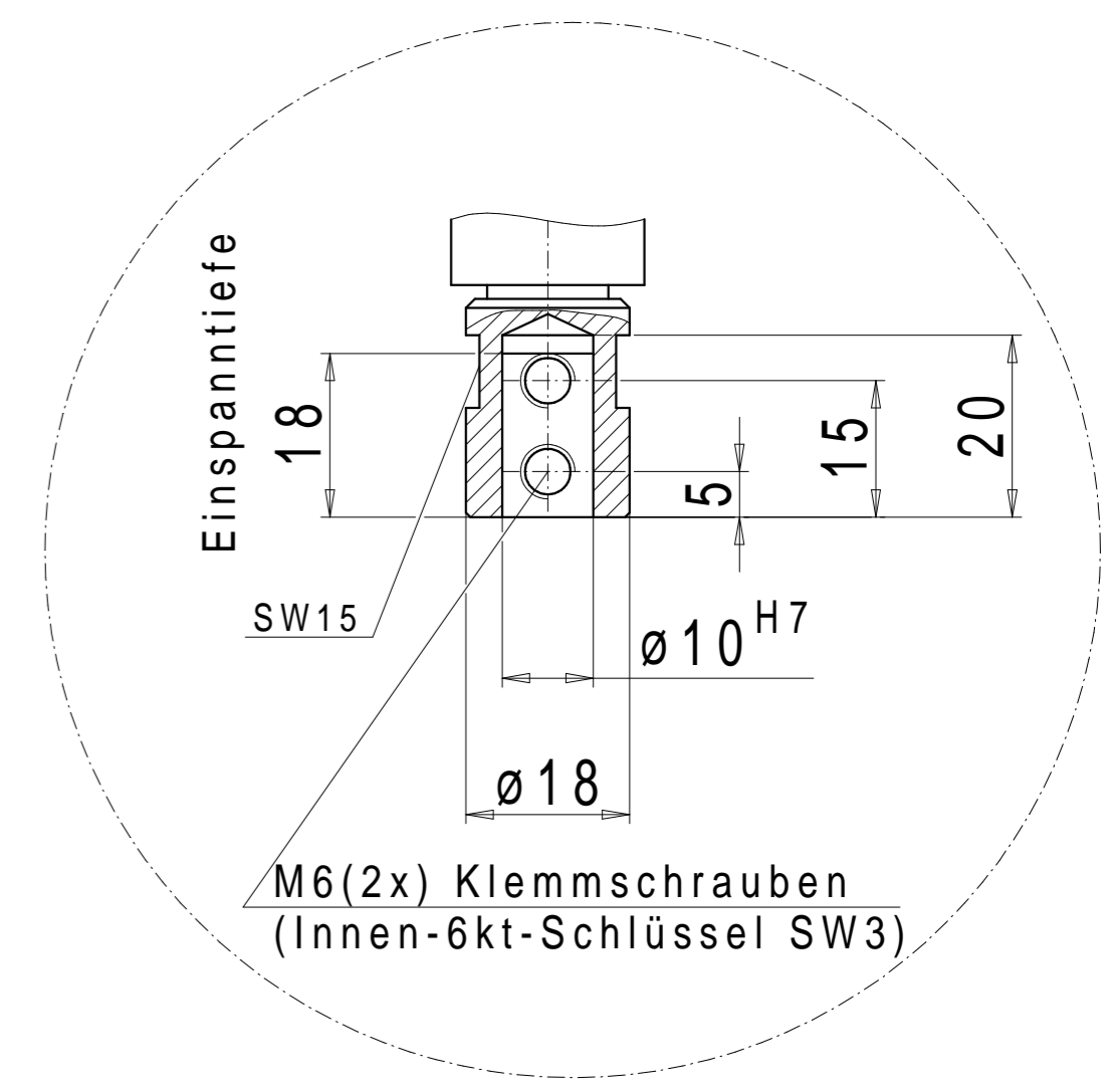
Schaftaufnahme \phi 10H7 RE
