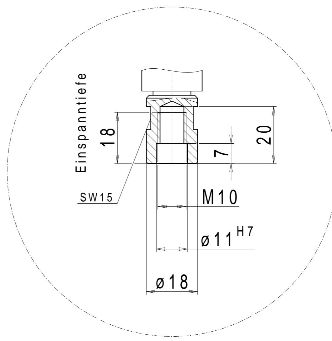
Schaftaufnahme M10 pl. RE
