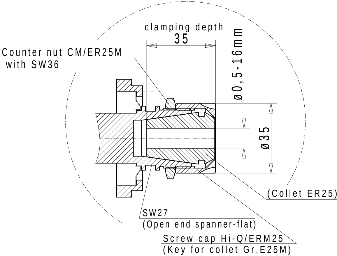
Collet receptacle Hi-Q/ERM25
