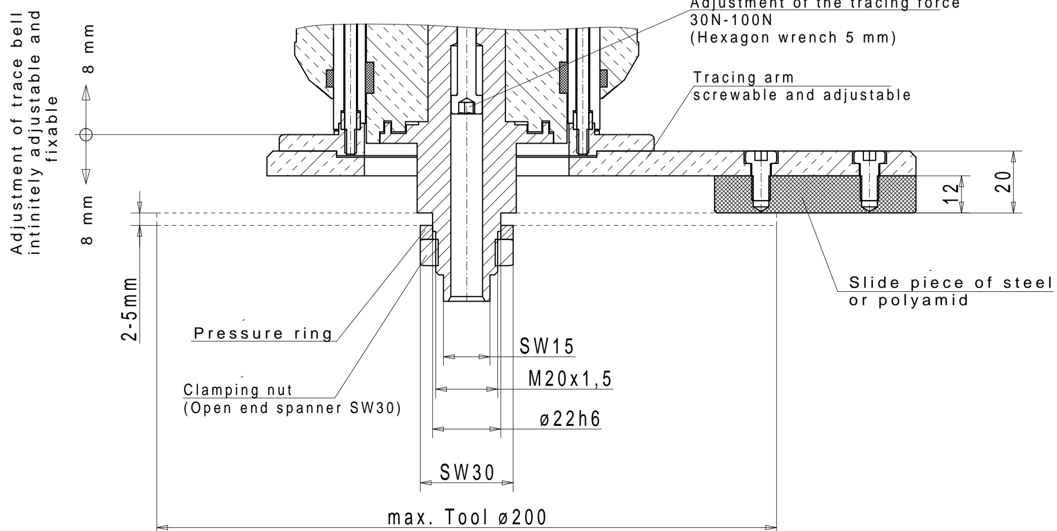
Tool receptacle
