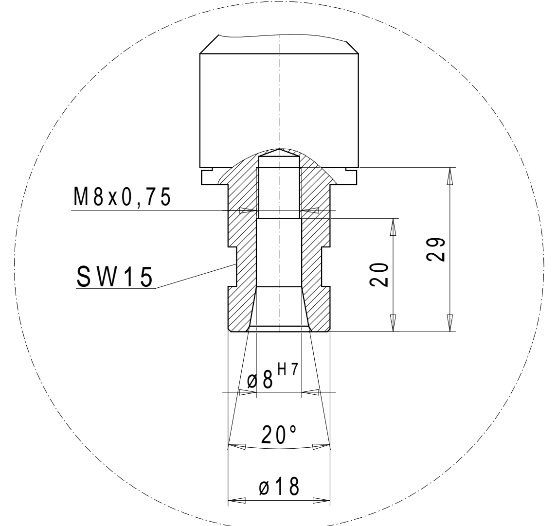
Collet receptacle 601E R.H./L.H.
