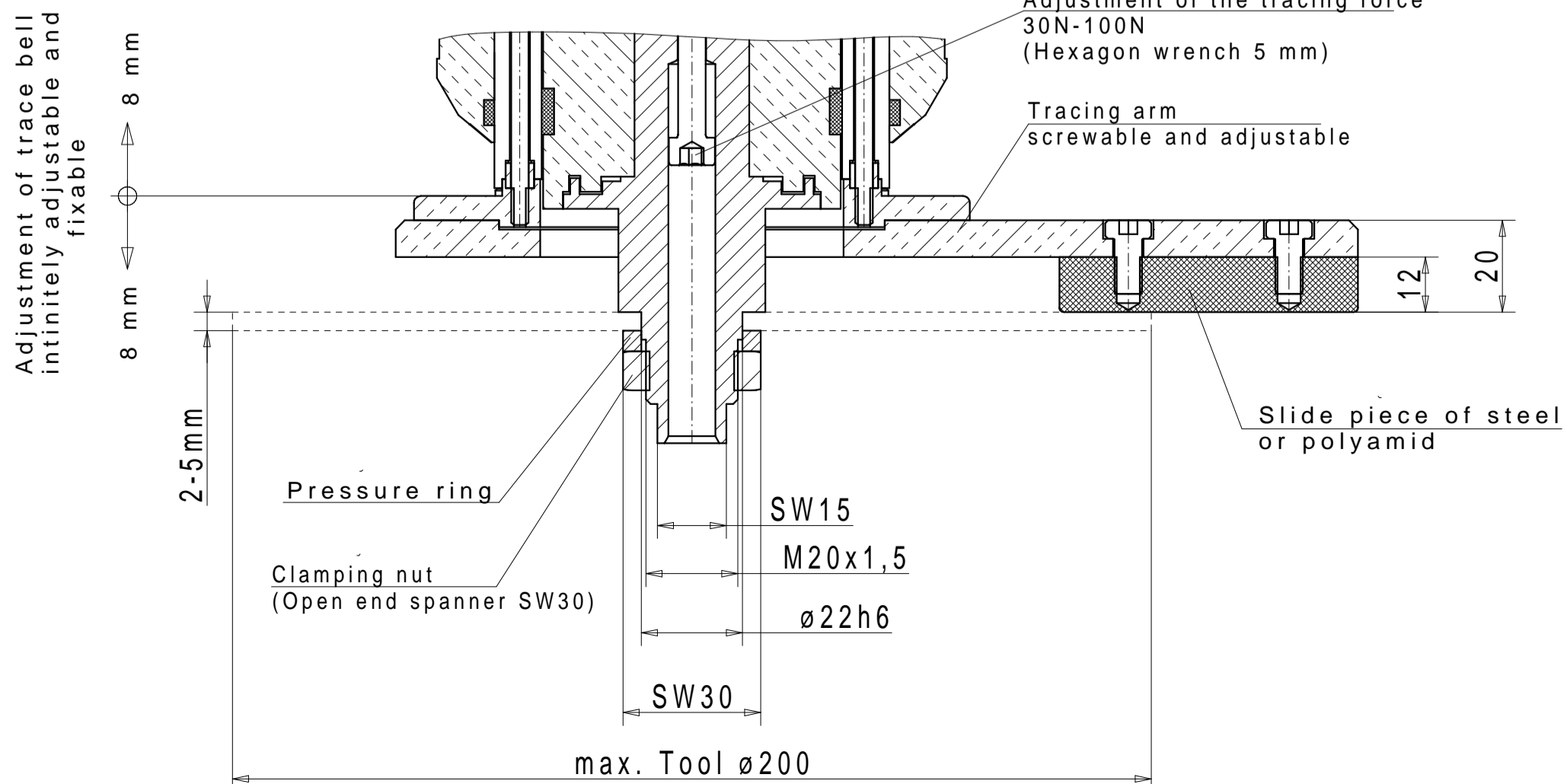
Tool receptacle
