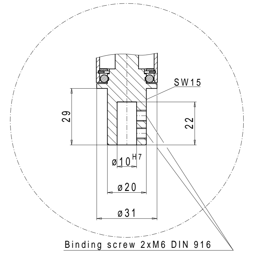
Shank receptacle \varnothing 10 \text{ H7-R.H./L.H.}
