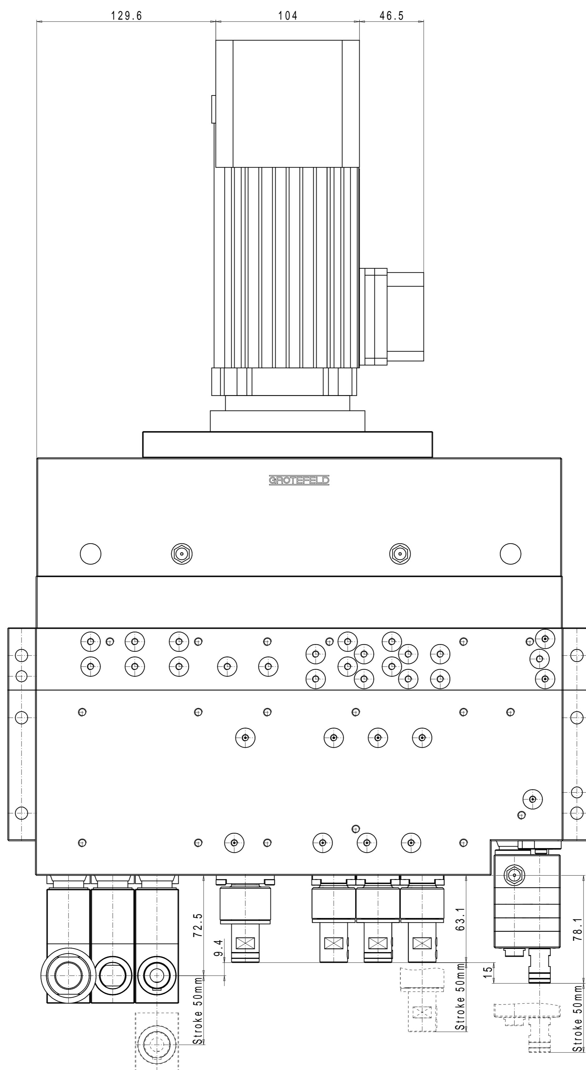
Vertical-Shank receptacle BGVT \varnothing 8 \text{ H7-R.H./L.H.}
