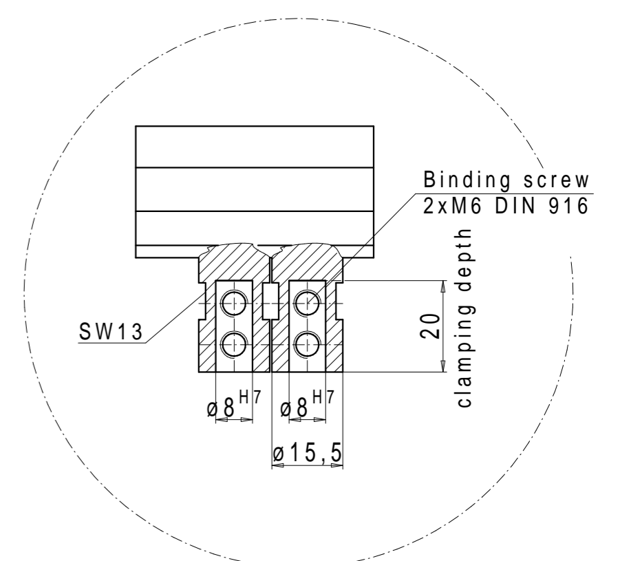
Vertical-Shank receptacle BGVT \varnothing 8 \text{ H7-R.H./L.H.}
