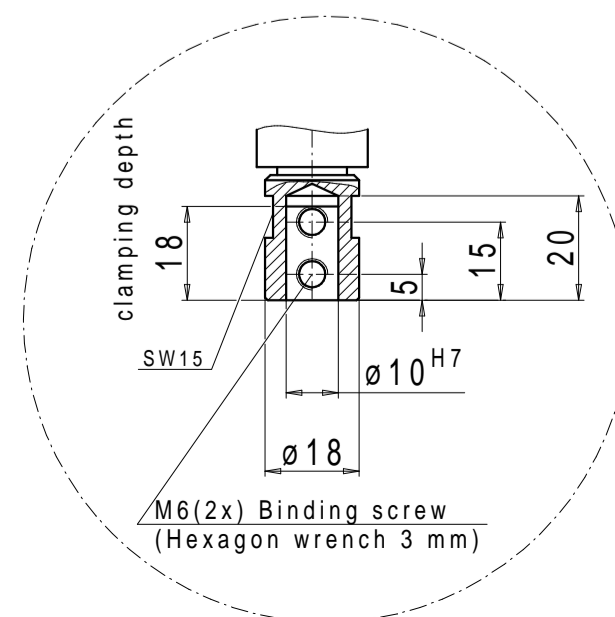
Shank receptacle \varnothing 10H7 R.H./L.H.
