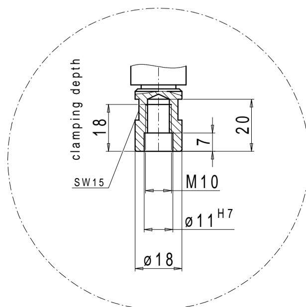
Shank receptacle M10 pl. R.H./L.H.
