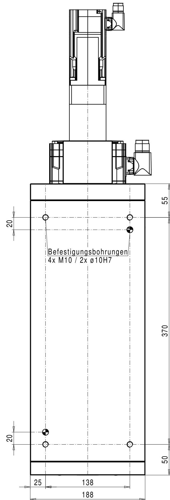
Einzelheit X Bohreraufnahme 10H7x20 zylindrisch mit 2 seitlichen M6 Klemmschrauben Artikelnummer 142001
