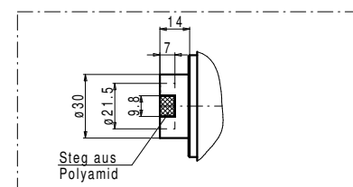
Antriebsstück (Kupplung) zum Antrieb von GROTEFELD-Mehrspindelbohrgetrieben Artikelnummer 143009
