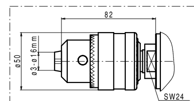
Zahnkranzbohrflutter von 3 mm bis max. 16 mm Artikelnummer 143005
